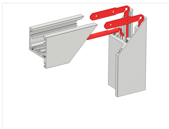
Alternative : raccord avec des cornières
