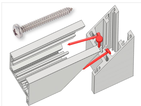
Raccord avec des vis
