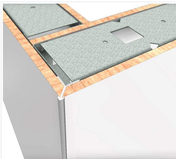
Option 1 : Angle extérieur en aluminium 5x5 mm
