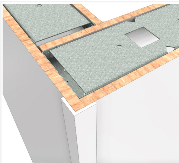
Option 2 : Angle extérieur en aluminium 20x20 mm.
